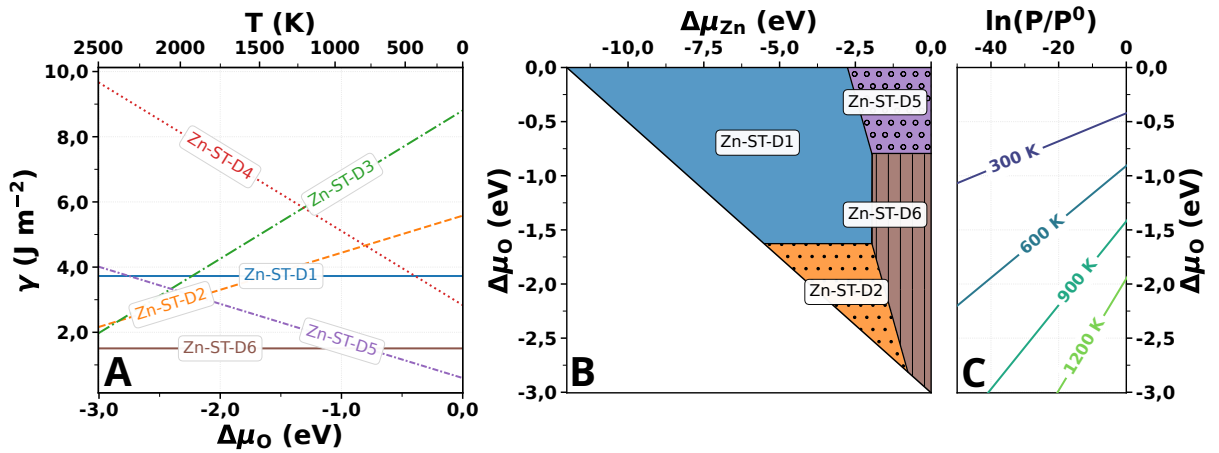
Figura 12: (A) \gamma em função de \Delta\mu_{\text{O}} para as diferentes terminações superficiais (100) do \text{ZnWO}_4 (B) Diagrama de estabilidade das terminações superficiais (100) em função de \Delta\mu_{\text{O}} e \Delta\mu_{\text{Zn}} . (C) Relação de T para diferentes \Delta\mu_{\text{O}} e pressões parciais de \text{O}_2 .
