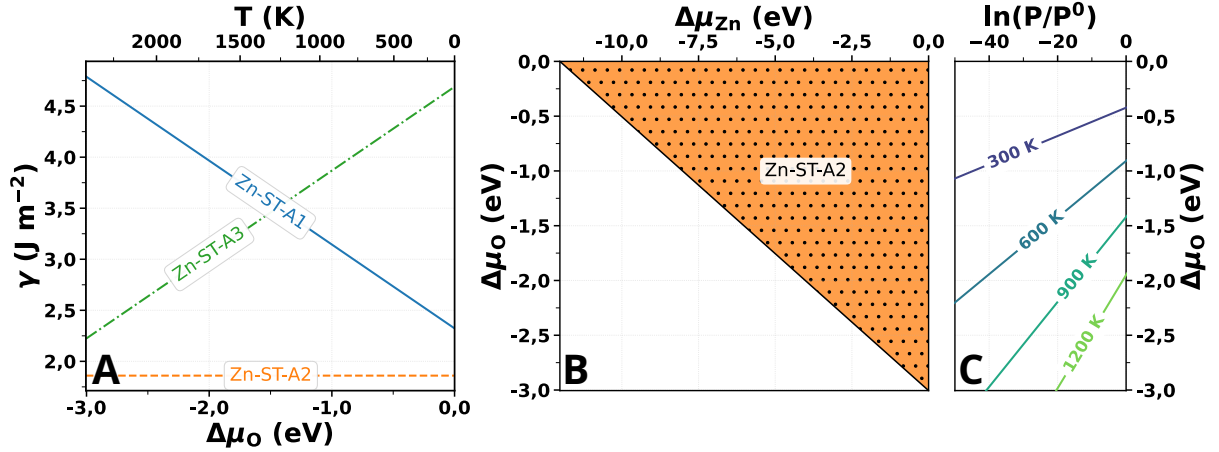
Figura 14: (A) \gamma em função de \Delta\mu_{\text{O}} para as diferentes terminações superficiais (101) do \text{ZnWO}_4 (B) Diagrama de estabilidade das terminações superficiais (101) em função de \Delta\mu_{\text{O}} e \Delta\mu_{\text{Zn}} . (C) Relação de T para diferentes \Delta\mu_{\text{O}} e pressões parciais de \text{O}_2 .
