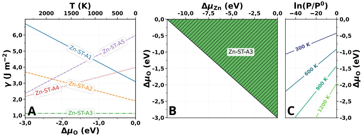
Figura 7: (A) \gamma em função de \Delta\mu_{\text{O}} para as diferentes terminações superficiais (001) do \text{ZnWO}_4 . (B) Diagrama de estabilidade das terminações superficiais (001) em função dos potenciais químicos do oxigênio \Delta\mu_{\text{O}} e \Delta\mu_{\text{Zn}} . (C) Relação de T para diferentes \Delta\mu_{\text{O}} e pressões parciais de \text{O}_2 .
